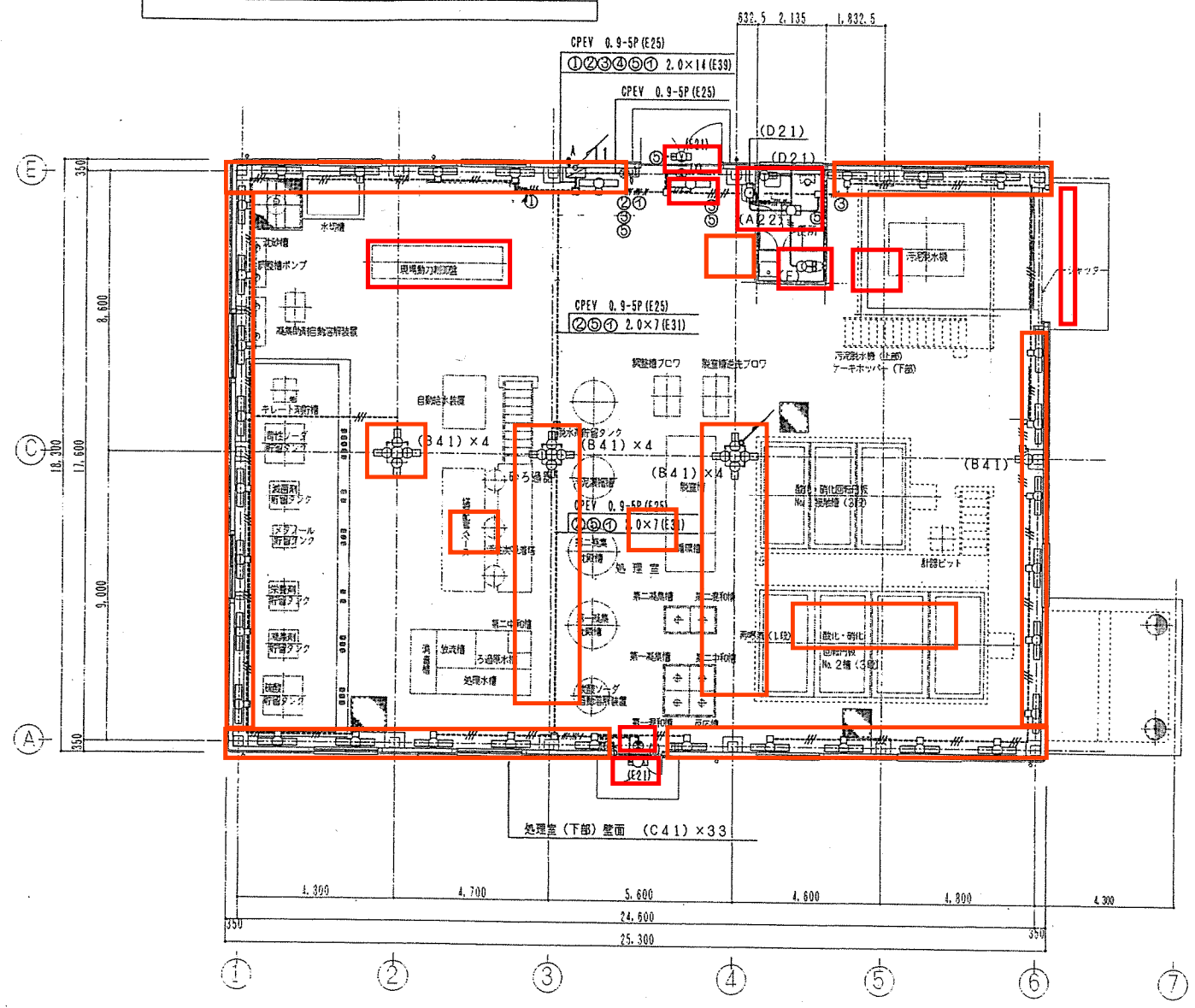
1階平面図 1:100
